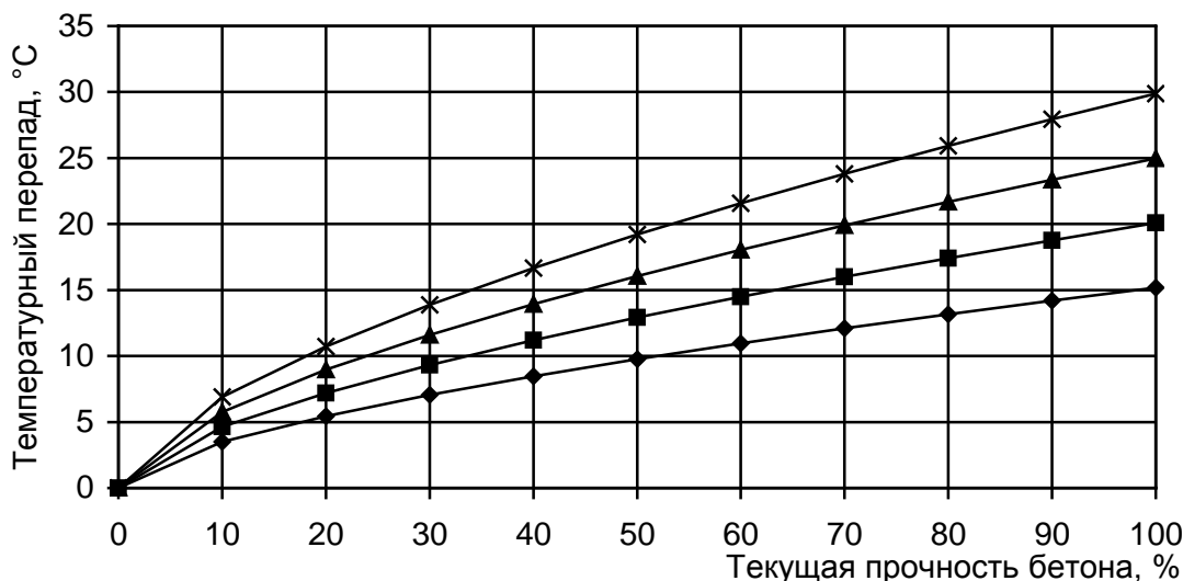
Рисунок 3. Максимальные температурный перепад по сечению конструкции
